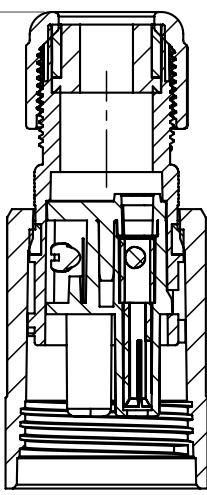
SEZIONE A-A
